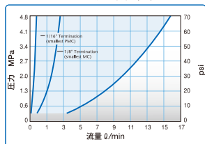
PMC12 流量特性 (水)
